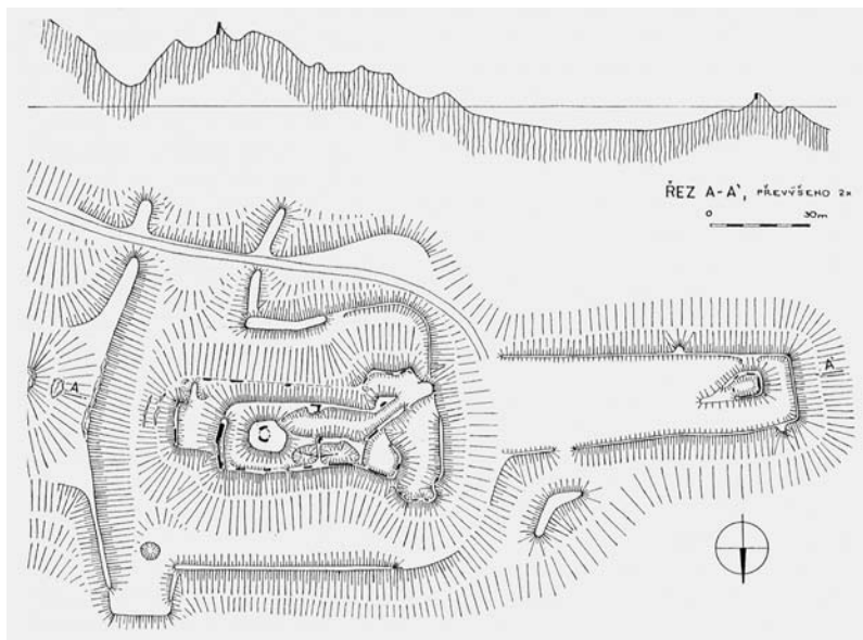
/ Hrad u Dobrušan, terénní náčrt půdorysu zříceniny.
